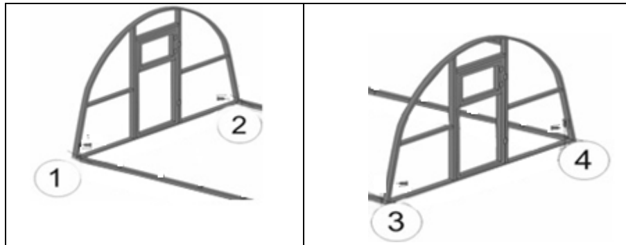
Pav. 9. Sujungimo vietas naudojant savisriegius varžtus (pozicija Nr. 1, 2, 3, 4). Jei šiltnamį tvirtinamas prie pamato, tvirtinimui naudojami savisriegiai varžtai (Pav. 10).
