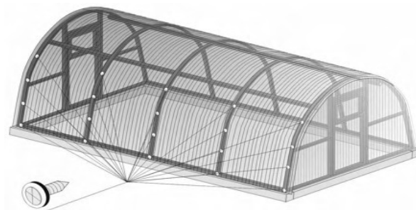
Pav. 10. Savisriėgių varžtų tvirtinimo mazgai šiltnamio viršutinėje dalyje
