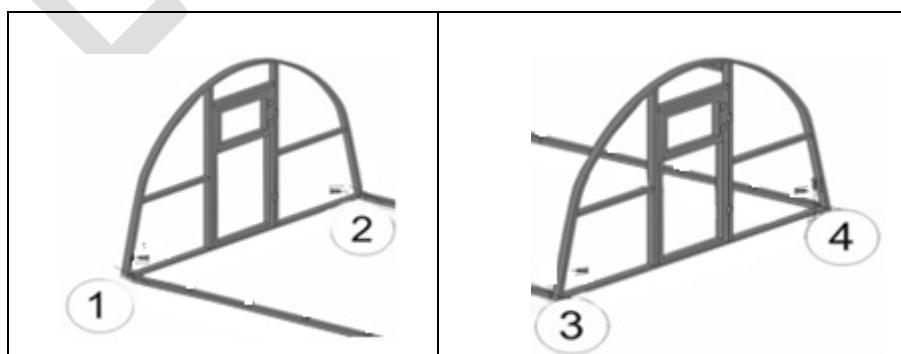
Pav. 9. Sujungimo vietos naudojant savisriegius varžtus (pozicija Nr. 1, 2, 3, 4). Jei šiltnamis tvirtinamas prie pamato, tvirtinimui naudojami savisriegiai varžtai (Pav. 10).
