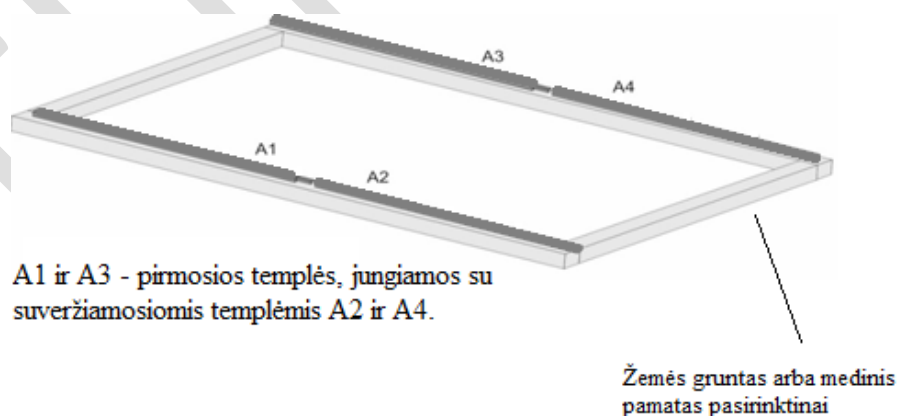
Pav. 6. Pirmųjų ir suveržiamųjų templių išdėstymas
