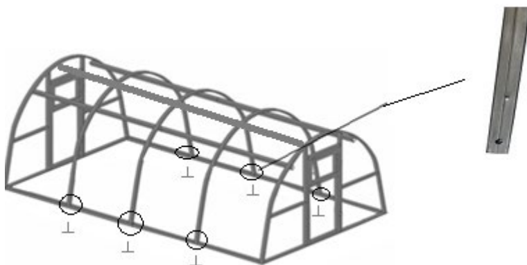
Pav. 11. Lankų tvirtinimas
