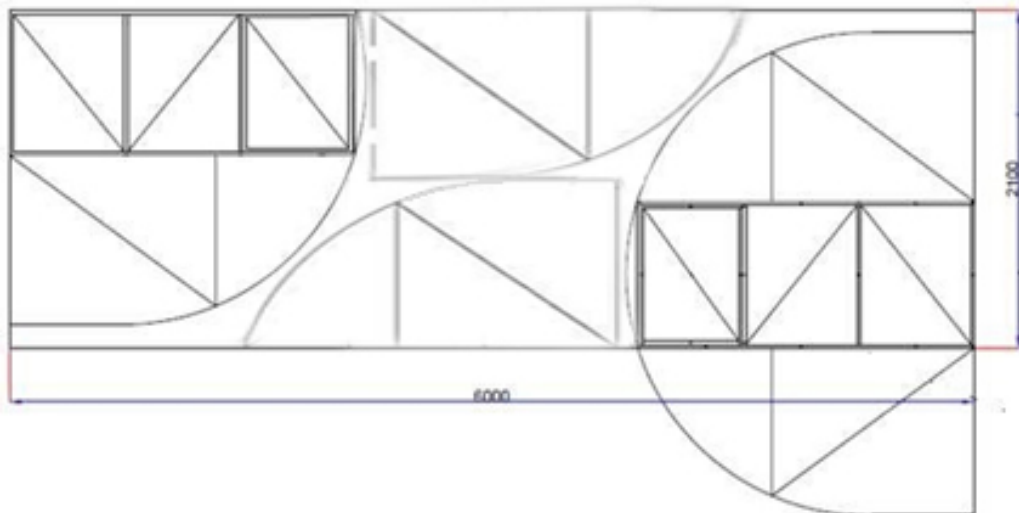
Pav. 1 Polikarbonato pjovimas
