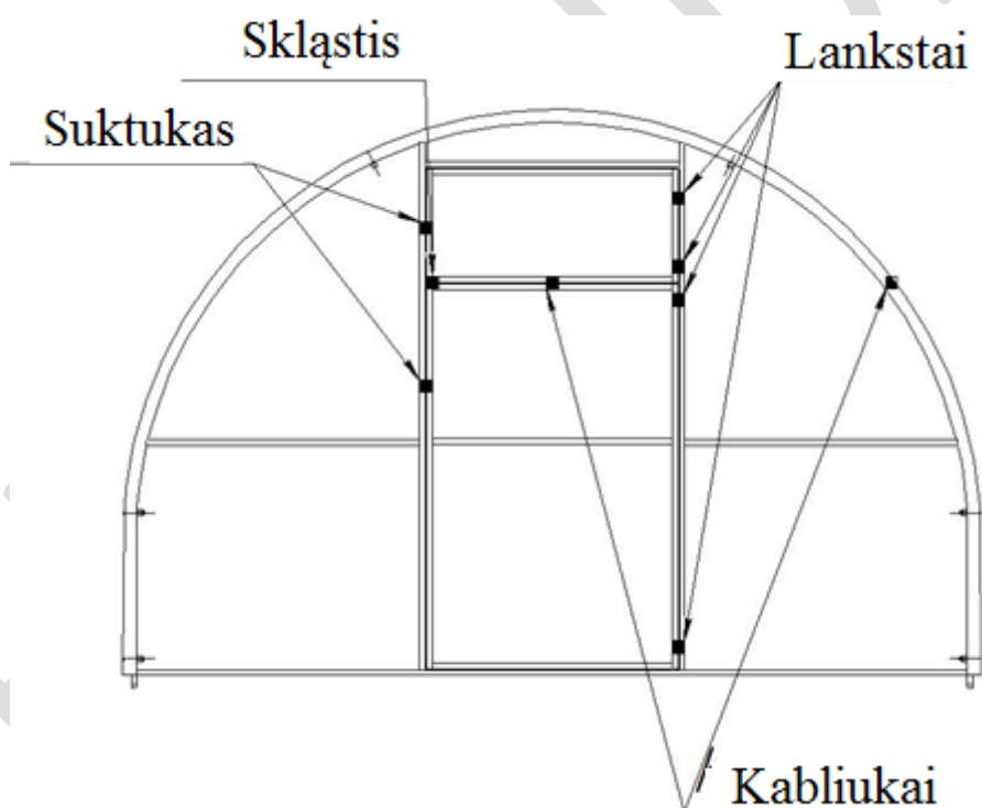
Pav. 16 Suktukų, skląsčių, lankstų, kabliukų tvirtinimo vietos
