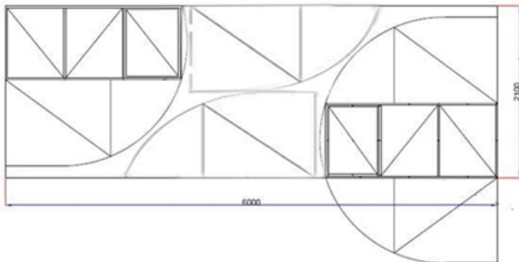
Pav. 2 Polikarbonato pjovimas
