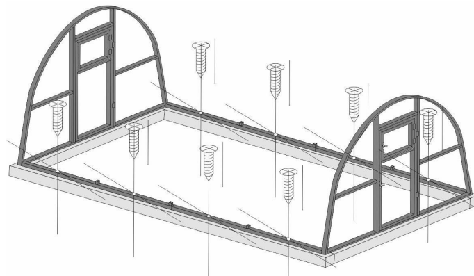
Pav. 12. Tvirtinimas prie pamato
