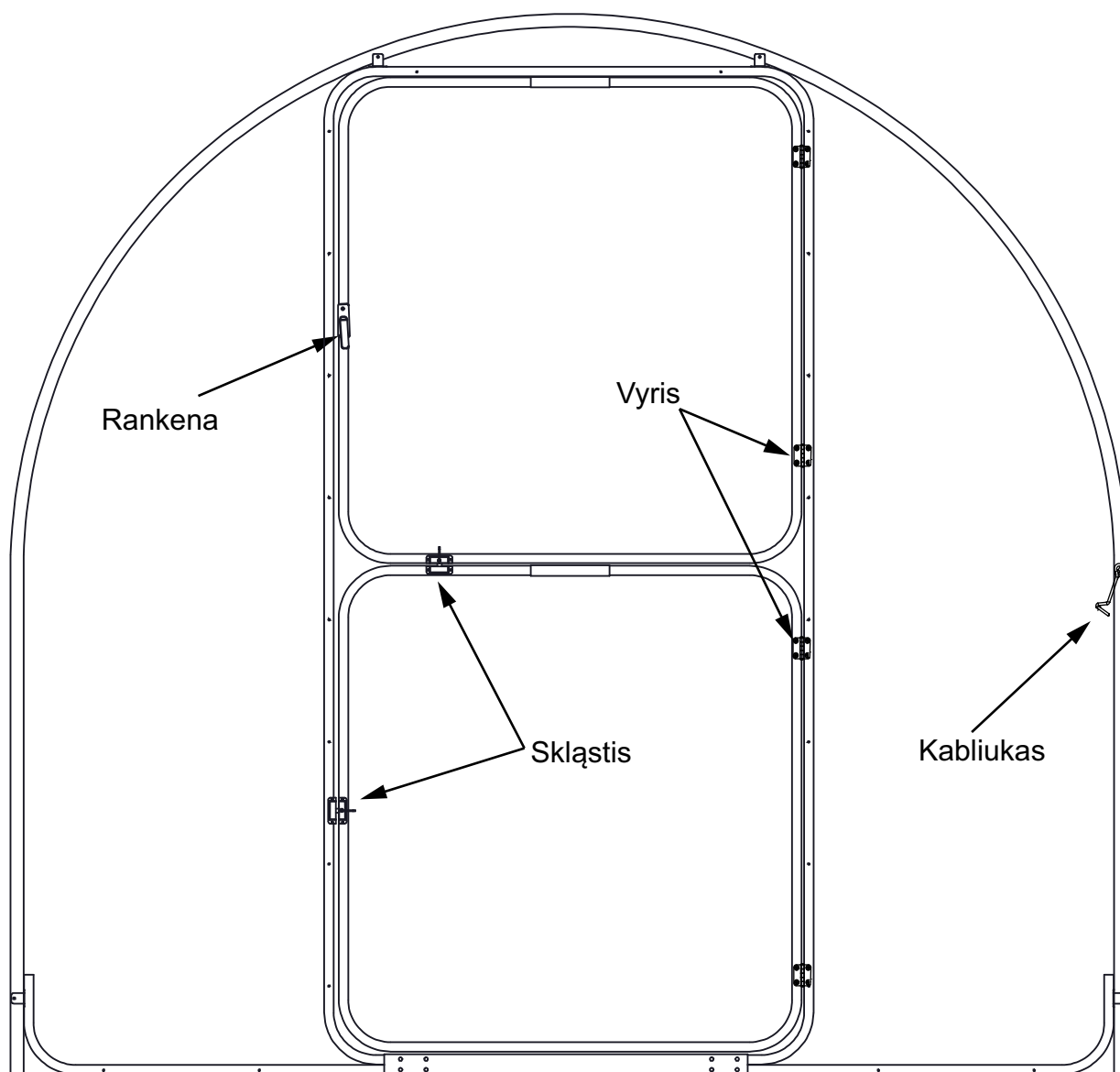
2 pav. - jungiamųjų detalių tvirtinimo schema
