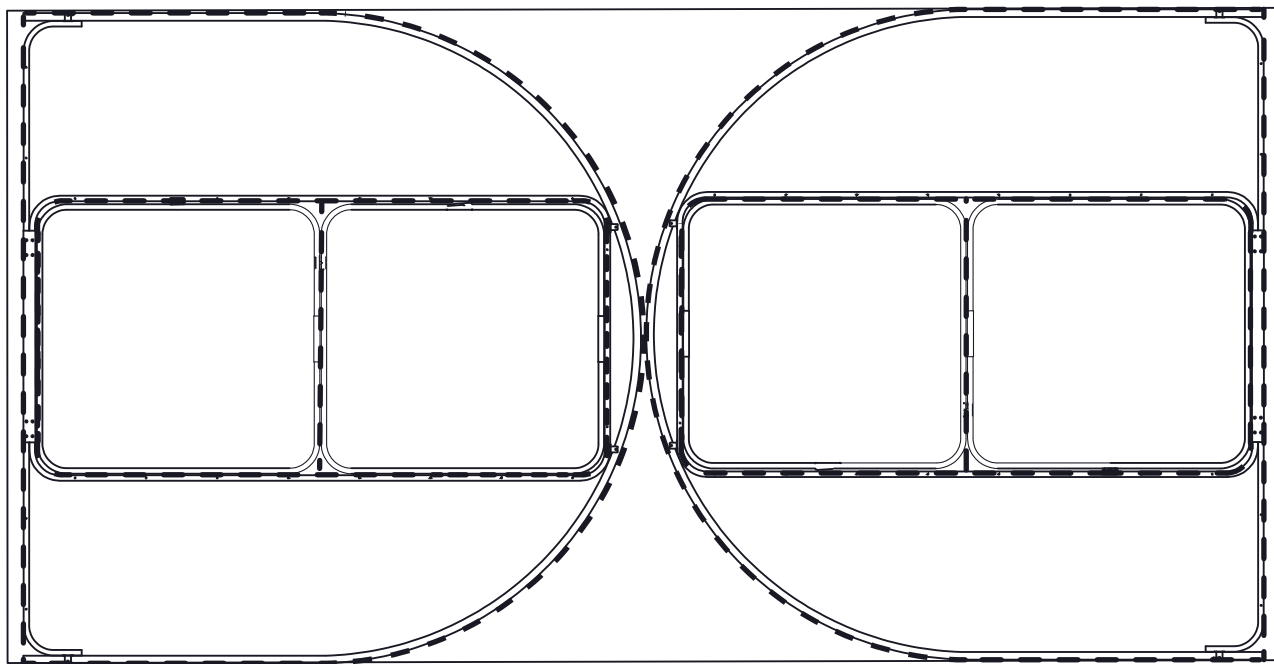
1 pav. Polikarbonato pjovimo schema
