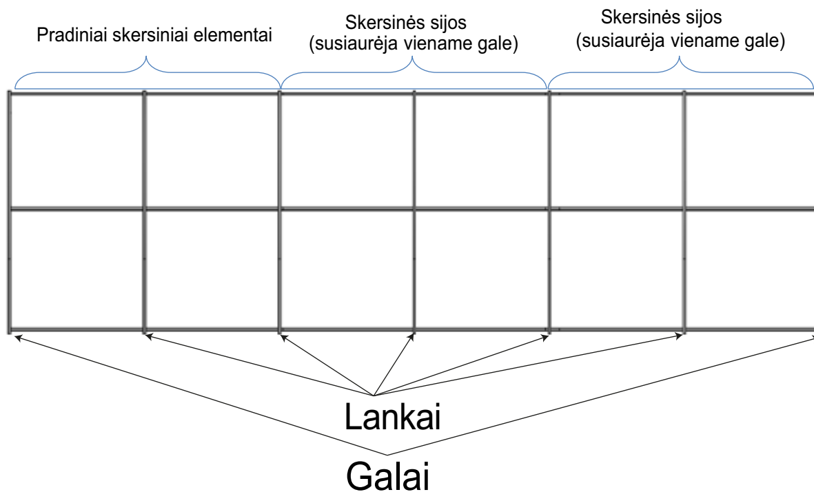
3 pav. - šiltnamio rėmo skersinių ir lankų tarpusavio padėtis (6 m ilgio šiltnamio pavyzdys, vaizdas iš šono)
