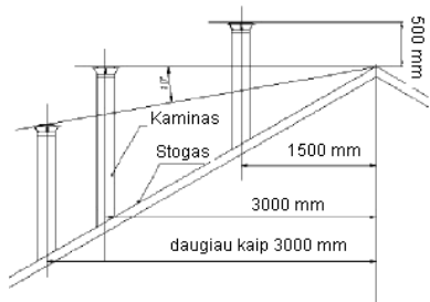
Pav. 1
