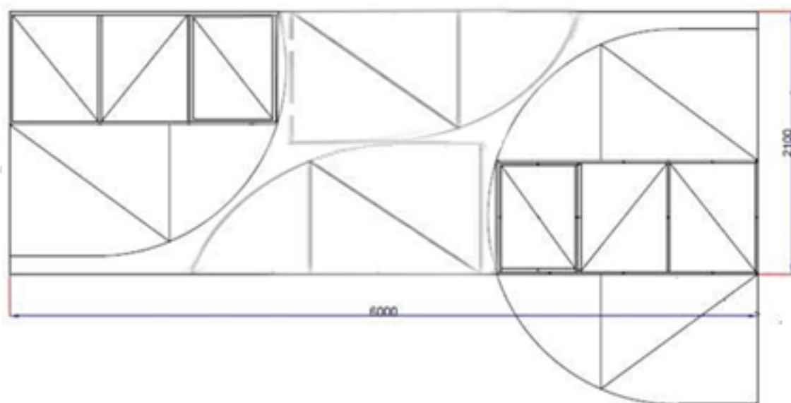
Pav. 22 Polikarbonato pjovimas
