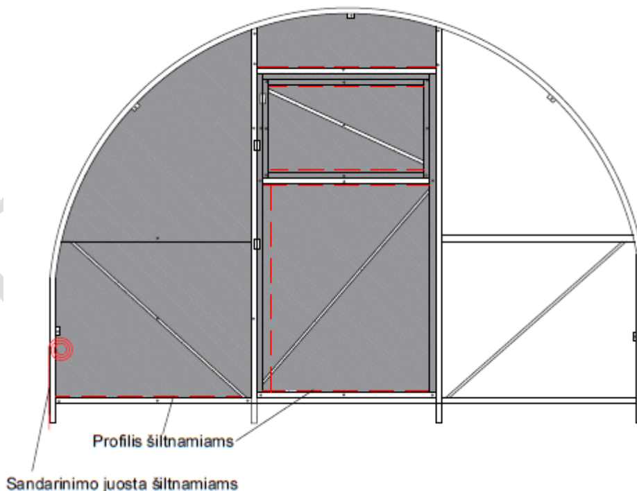
Pav. 24 Polikarbonato dangos montavimas ant šiltnamio rėmo
