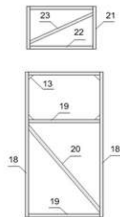
Pav. 5. durys ir orlaidė
