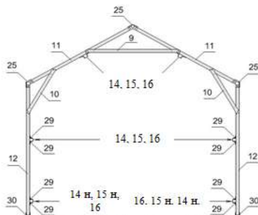
Pav. 3. tarpinė šiltnamio konstrukcija
